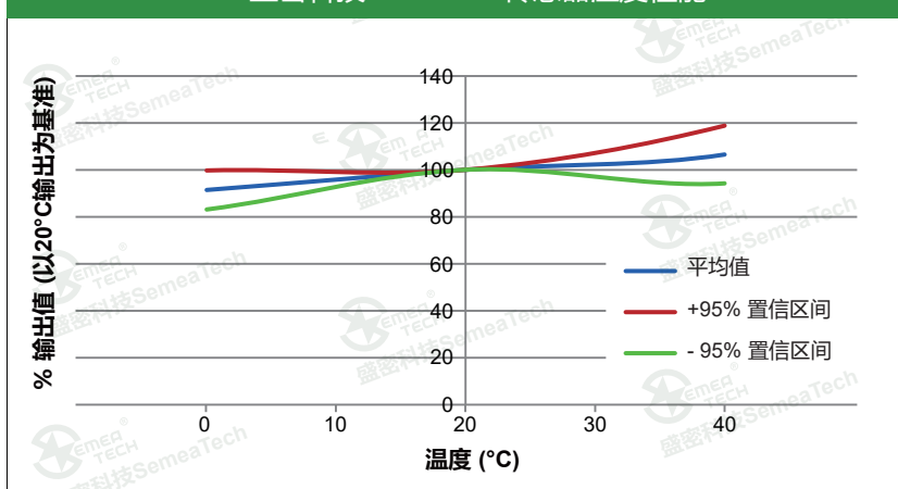
盛密科技4SM HF-5传感器温度性能
